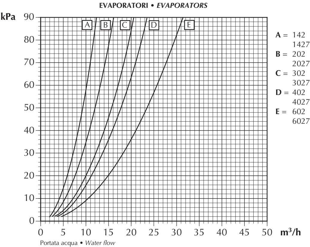
TAV 1 PERDITE DI CARICO • PRESSURE DROPS
