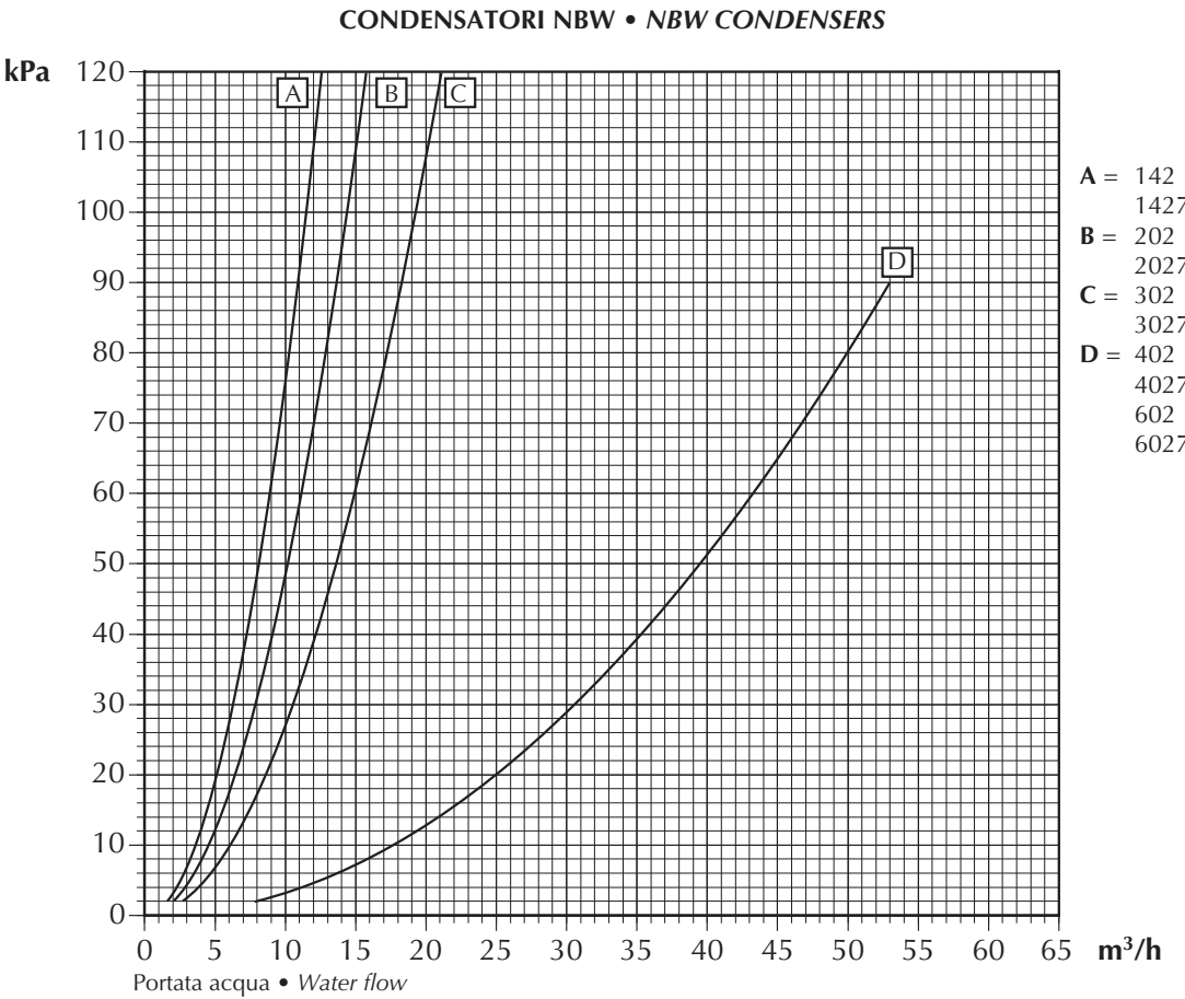
TAV 2 PERDITE DI CARICO • PRESSURE DROPS
