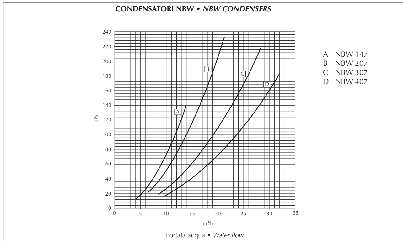
TAV 10 PERDITE DI CARICO • PRESSURE DROPS
