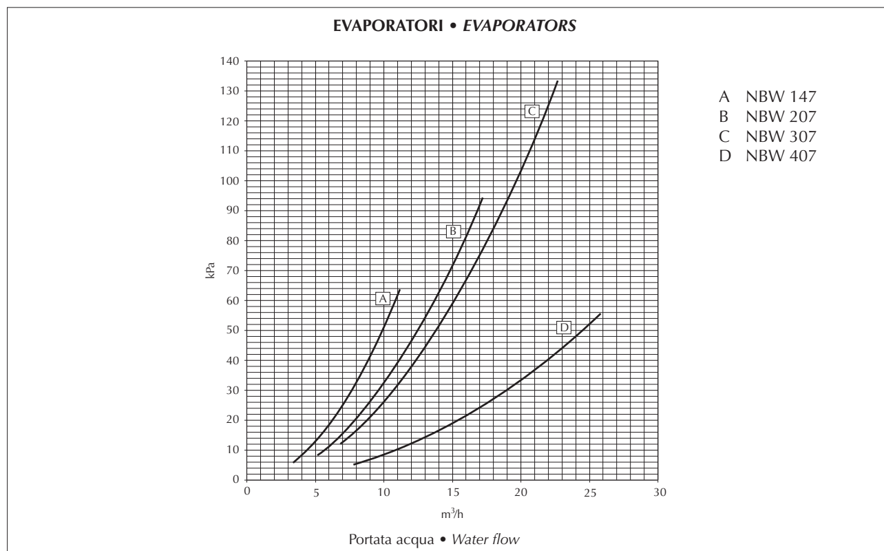
TAV 10 PERDITE DI CARICO • PRESSURE DROPS
